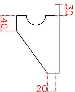
Piastra laterale finita
