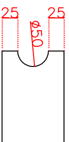
Particolare piastre 2-3 lavorate
