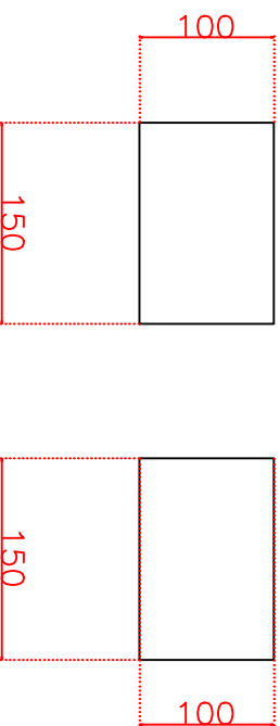
Piastra 2-3 spessore 8mm
